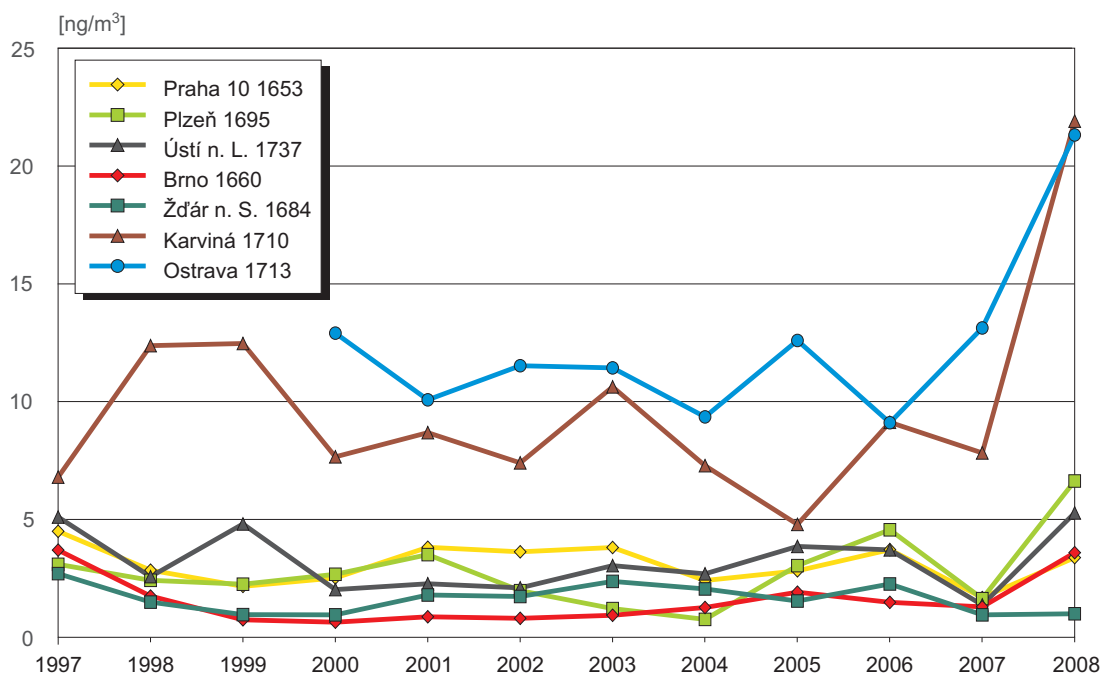
Obr. 2.4c Polycyklické aromatické uhlovodíky – hodnota toxického ekvivalentu benzo[a]pyrenu, 1997–2008 Fig. 2.4c Polycyclic aromatic hydrocarbons – Benzo[a]pyrene Toxic Equivalent TEQ, 1997–2008
