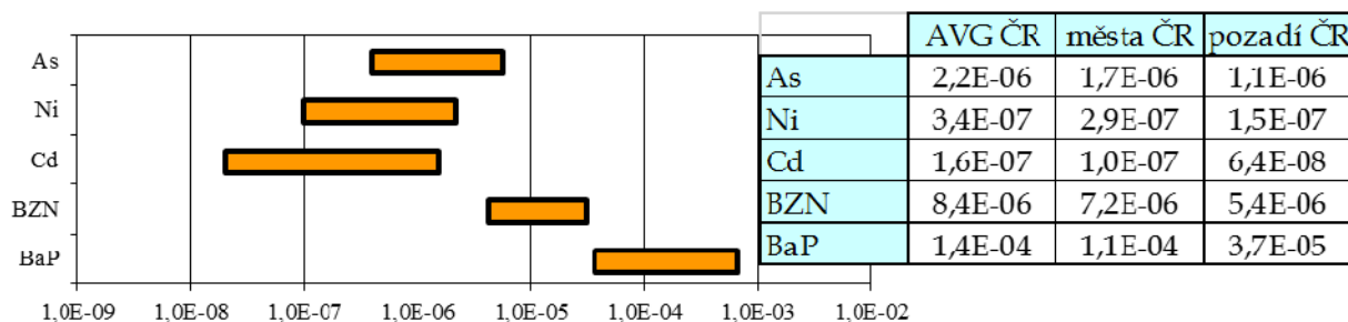
2018 - Průměr za ČR a rozpětí odhadu pravděpodobnosti zvýšení počtu nádorových onemocnění (ILCR) z příjmu As, Ni, Cd, benzenu a BaP z venkovního ovzduší
