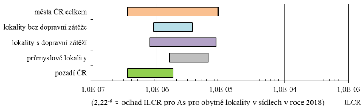
Rozpětí hodnot odhadu zdravotních rizik (ILCR) pro As v roce 2018 (ČR a jednotlivé typy městských lokalit)
