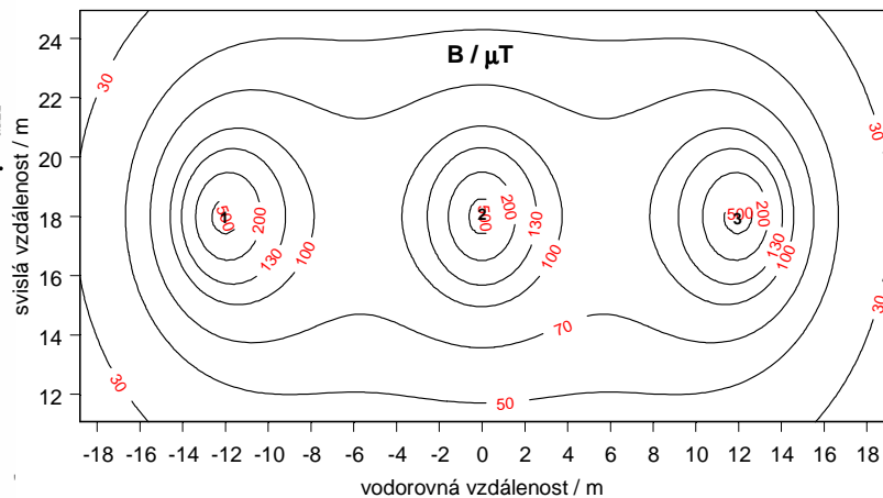
Obr. 10: Prostorové rozložení efektivní hodnoty velikosti magnetické indukce v okolí vodičů 400 kV, proud v jedné fázi = 2100 A
